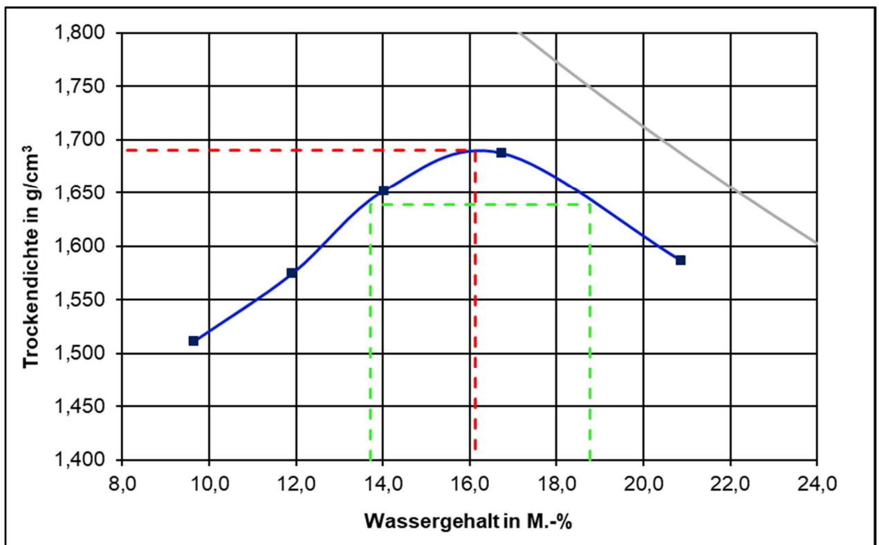
Proctorkurve der untersuchten HMV-Asche 0/32 (aus Prüfbericht F 22/08/0773 – III/2022)
