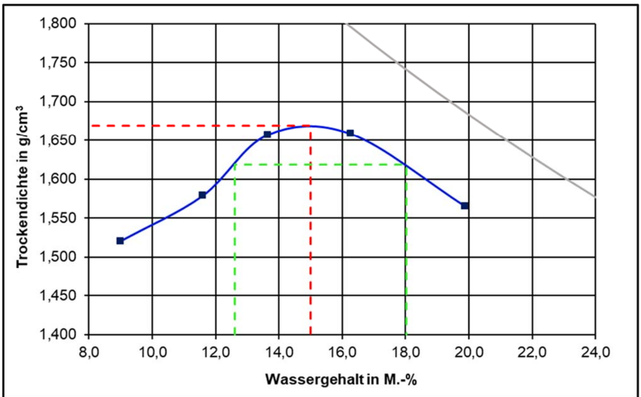
Proctorkurve der untersuchten HMV-Asche 0/32 (aus Prüfbericht F 21/08/0745 – III/2021)
