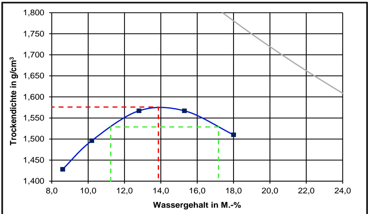
Proctorkurve der untersuchten HMV-Asche 0/32 (aus Prüfbericht F 20/07/0668 – III/2020)
