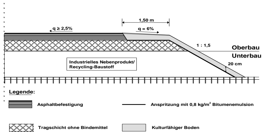
Bild 1: Damm, Anspritzung mit Bitumenemulsion und Abdeckung mit kulturfähigem Boden
