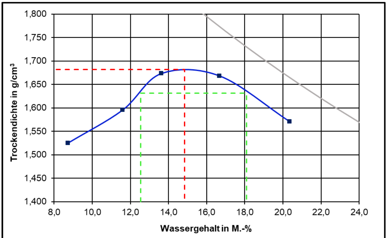
Proctorkurve der untersuchten HMV-Asche 0/32 (aus Prüfbericht F 22/03/0214 – I/2022)
