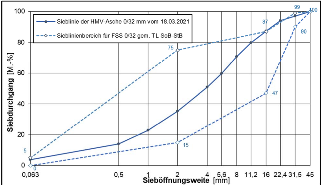
Korngrößenverteilung der untersuchten HMV-Asche 0/32 mm mit Anforderungen für Frostschuttschichten 0/32 mm gemäß TL SoB-StB /7/
