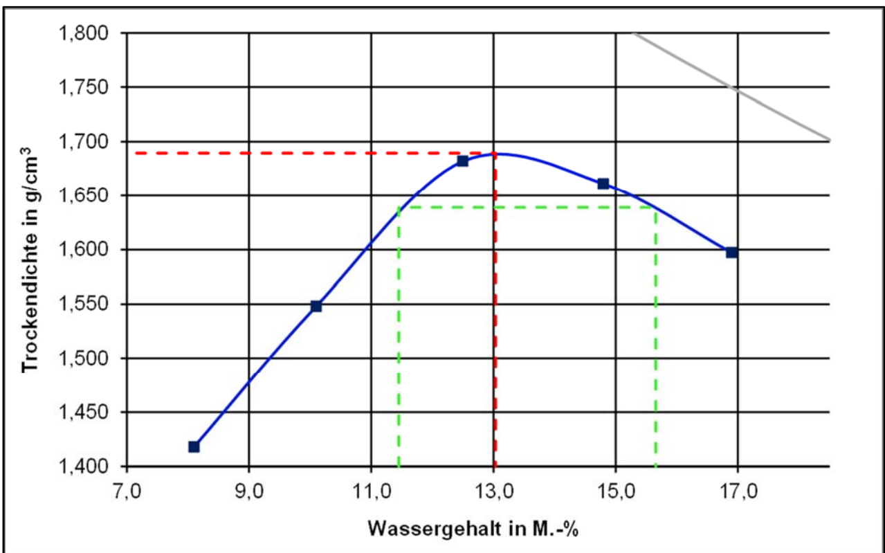
Proctorkurve der untersuchten HMV-Asche 0/32 (aus Prüfbericht F 21/02/0133 – I/2021)
