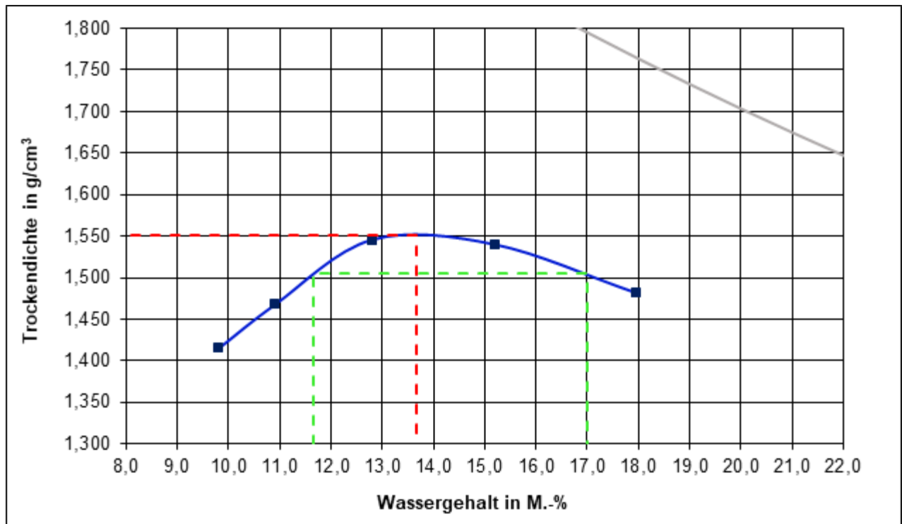
Proctorkurve der untersuchten HMV-Asche 0/32 (aus Prüfbericht F 20/02/0107 – I/2020)
