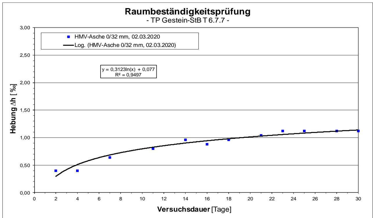
Abbildung 1: Verlauf der Hebung in Abhängigkeit von der Versuchsdauer der untersuchten HMV-Asche 0/32
