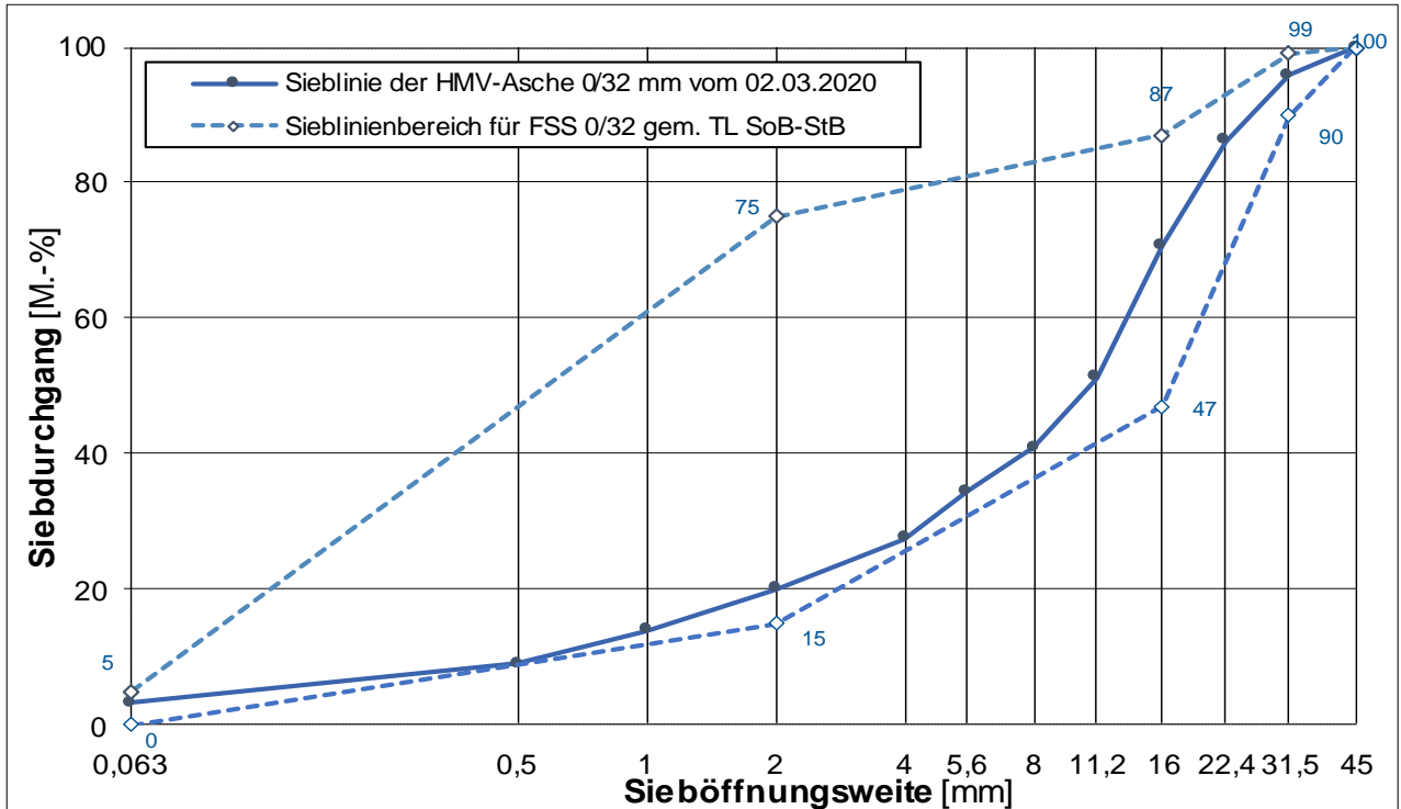
Korngrößenverteilung der untersuchten HMV-Asche 0/32 mit Anforderungen für Frostschuttschichten 0/32 mm gemäß TL SoB-StB /7/
