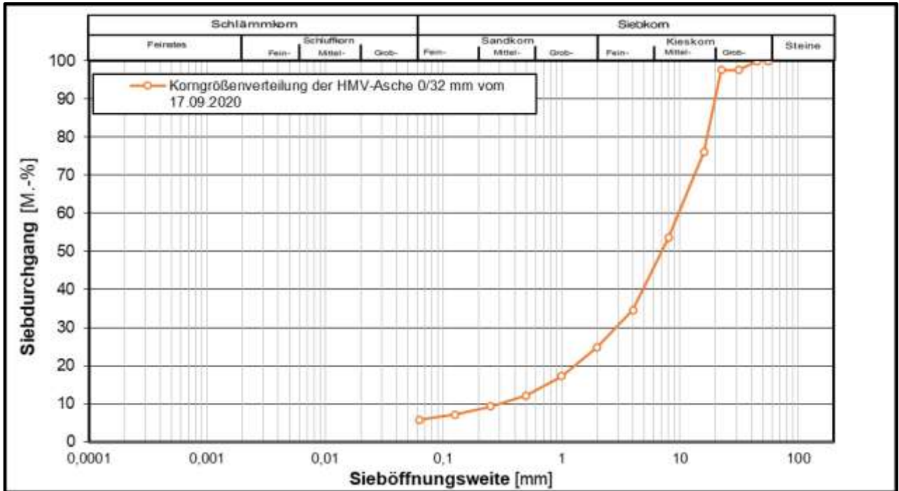
Korngrößenverteilung der untersuchten HMV-Asche 0/32
