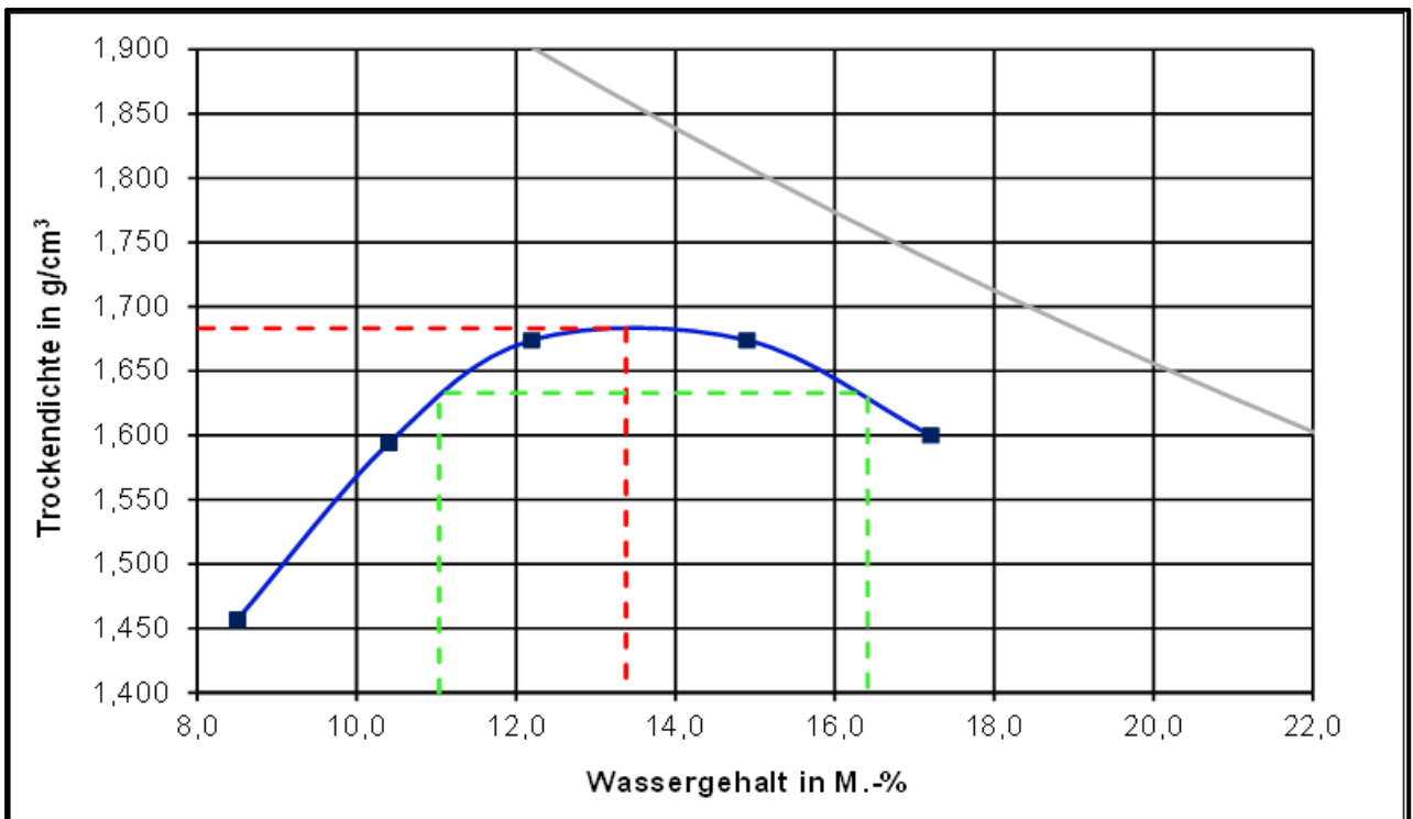
Proctorkurve der untersuchten HMV-Asche 0/32 (aus Prüfbericht F 20/07/0683)
