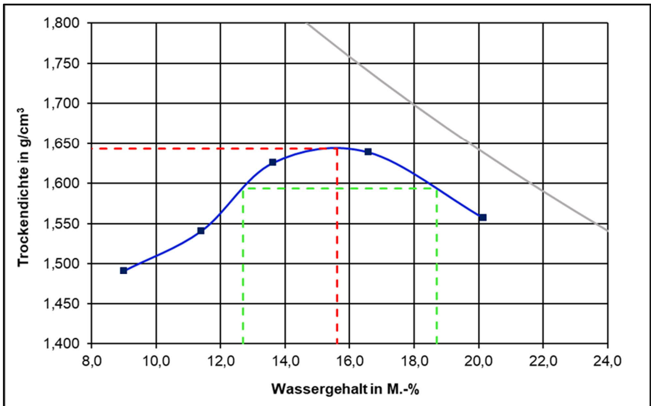
Proctorkurve der untersuchten HMV-Asche 0/32 (aus Prüfbericht F 21/09/0810)
