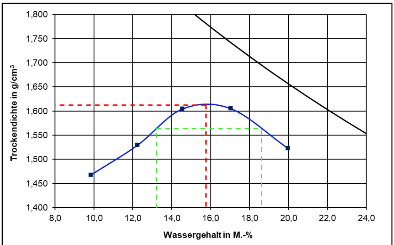
Proctorkurve der untersuchten HMV-Asche 0/32 (aus Prüfbericht F 21/03/0245)
