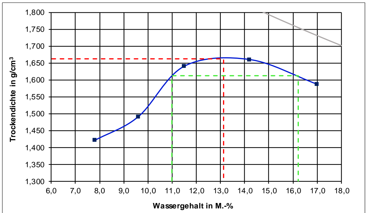
Proctorkurve der untersuchten HMV-Asche 0/32 (aus Prüfbericht F 20/02/0106)
