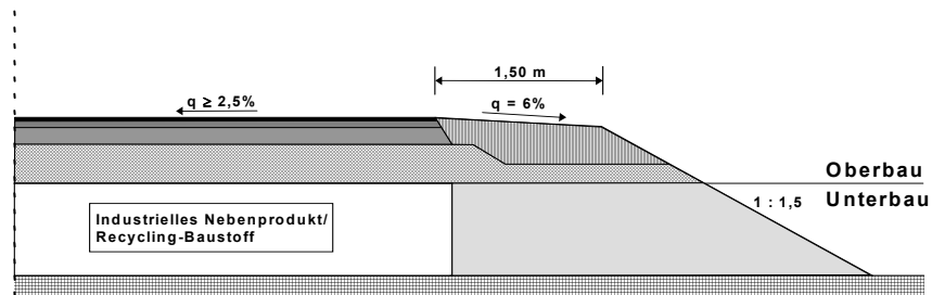
Bild 1: Damm, Anspritzung mit Bitumenemulsion und Abdeckung mit kulturfähigem Boden
