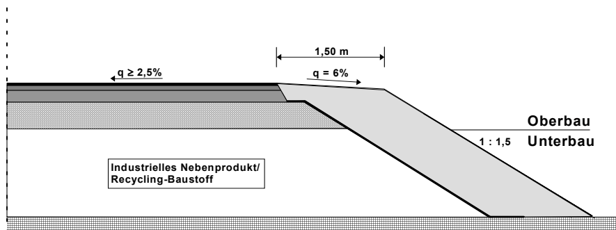
Bild 2: Damm, Abdeckung mit natürlichem/kulturfähigem Boden
