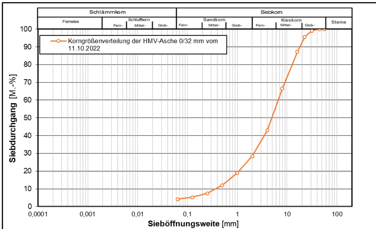
Korngrößenverteilung der untersuchten HMV-Asche 0/32
