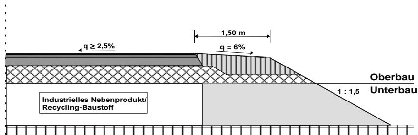
Bild 1: Damm, Anspritzung mit Bitumenemulsion und Abdeckung mit kulturfähigem Boden
