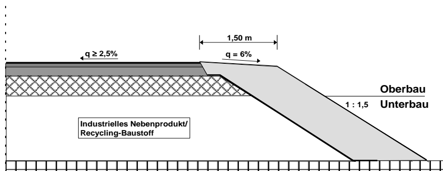
Bild 2: Damm, Abdeckung mit natürlichem/kulturfähigem Boden
