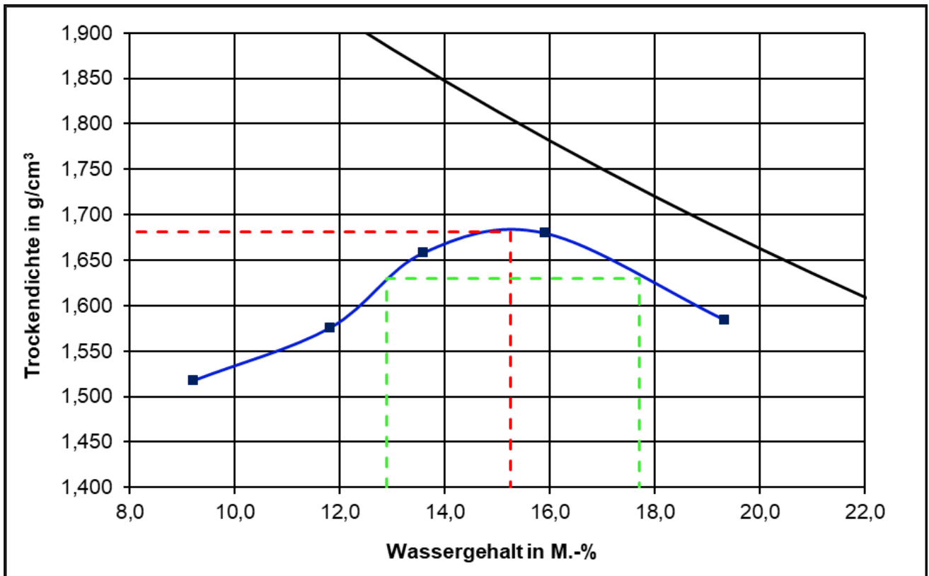
Proctorkurve der untersuchten HMV-Asche 0/32 (aus Prüfbericht F 21/03/0244)
