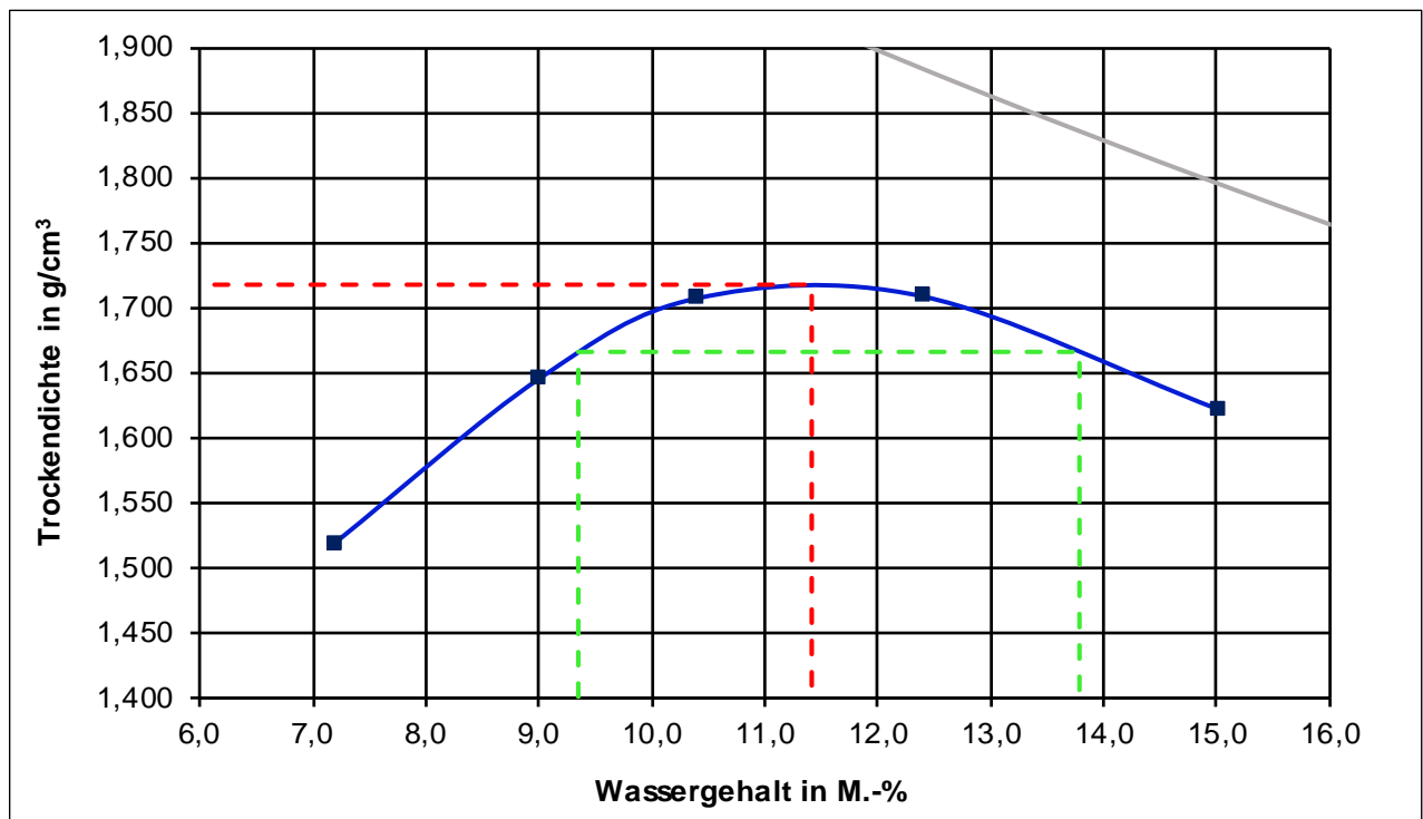
Proctorkurve der untersuchten HMV-Asche 0/32 (aus Prüfbericht F 20/02/0105)
