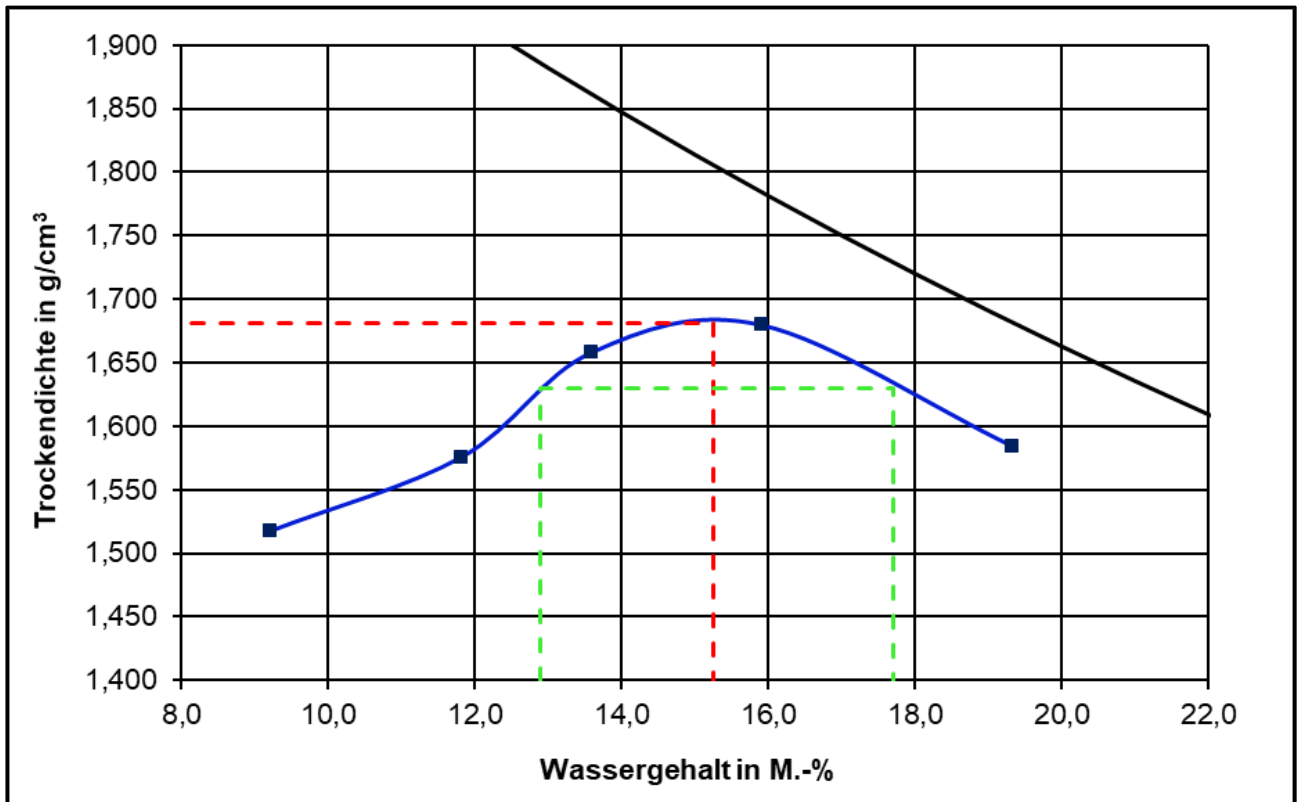
Proctorkurve der untersuchten HMV-Asche 0/32
