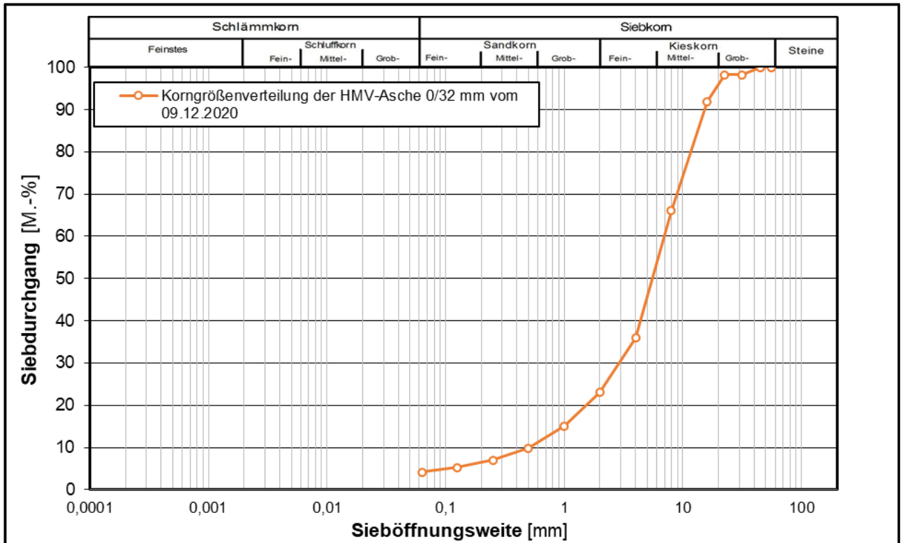
Korngrößenverteilung der untersuchten HMV-Asche 0/32
