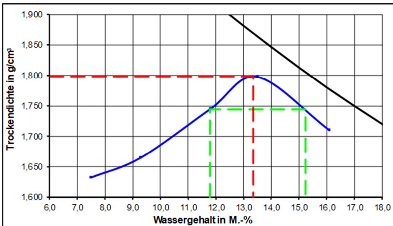
Proctorkurve der untersuchten HMV-Asche 0/32 (aus Prüfbericht F 18/07/0721 – III/2018)
