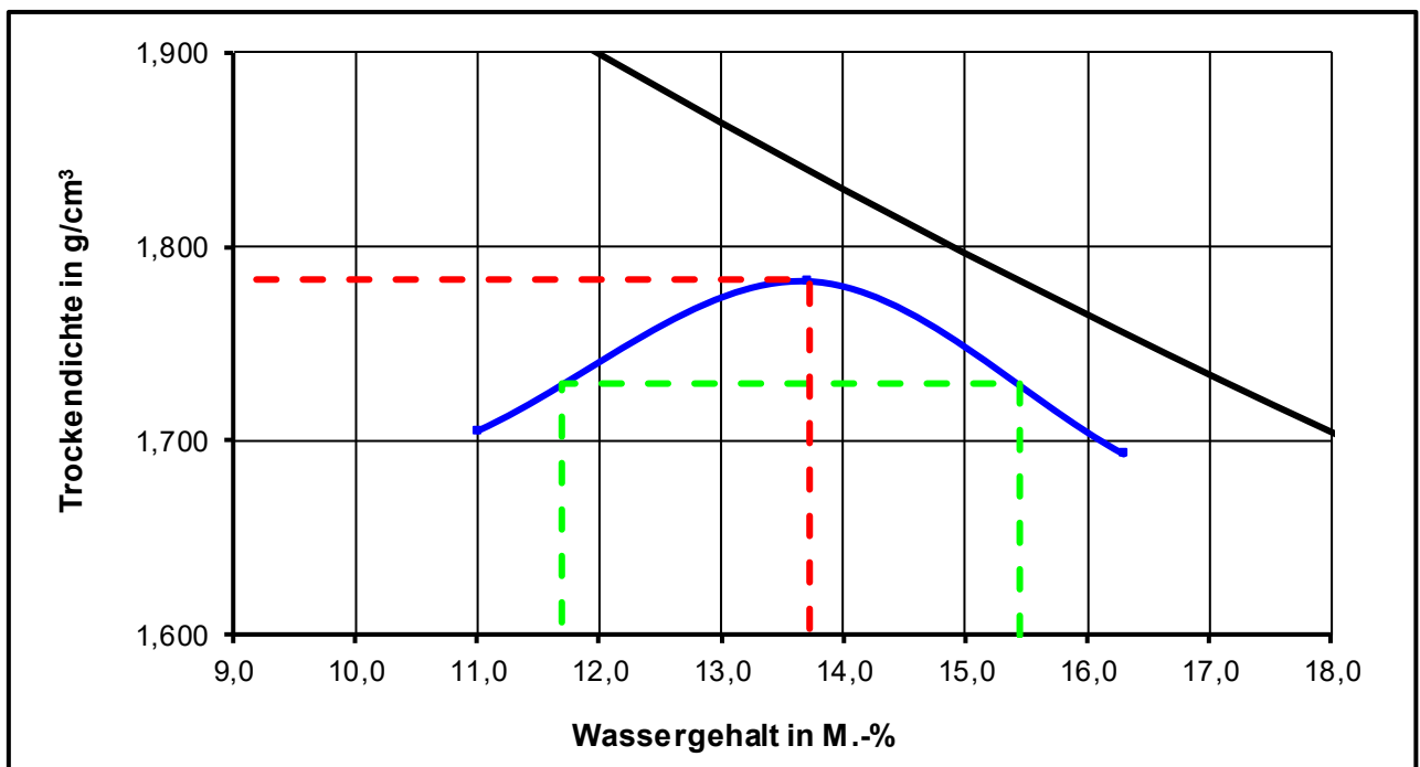
Proctorkurve der untersuchten HMV-Asche 0/32
