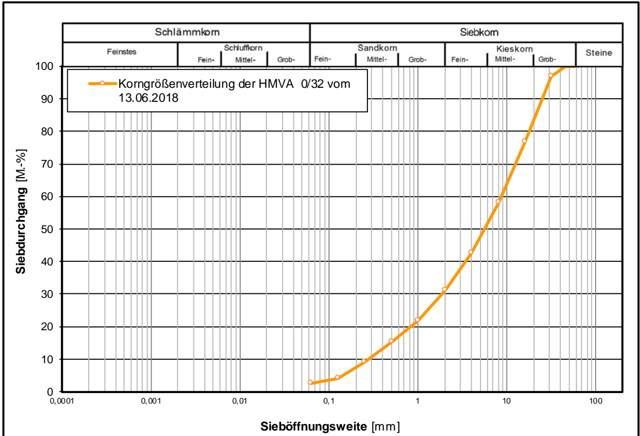
Korngößenverteilung der untersuchten HMV-Asche 0/32
