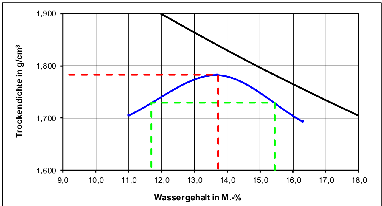
Proctorkurve der untersuchten HMV-Asche 0/32 (aus Prüfbericht F 18/08/0756)
