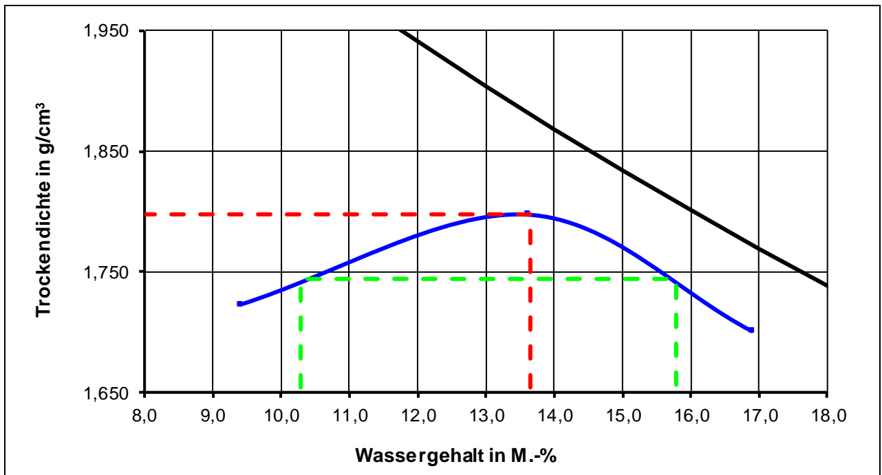
Proctorkurve der untersuchten HMV-Asche 0/32 (aus Prüfbericht F 18/08/0748)
