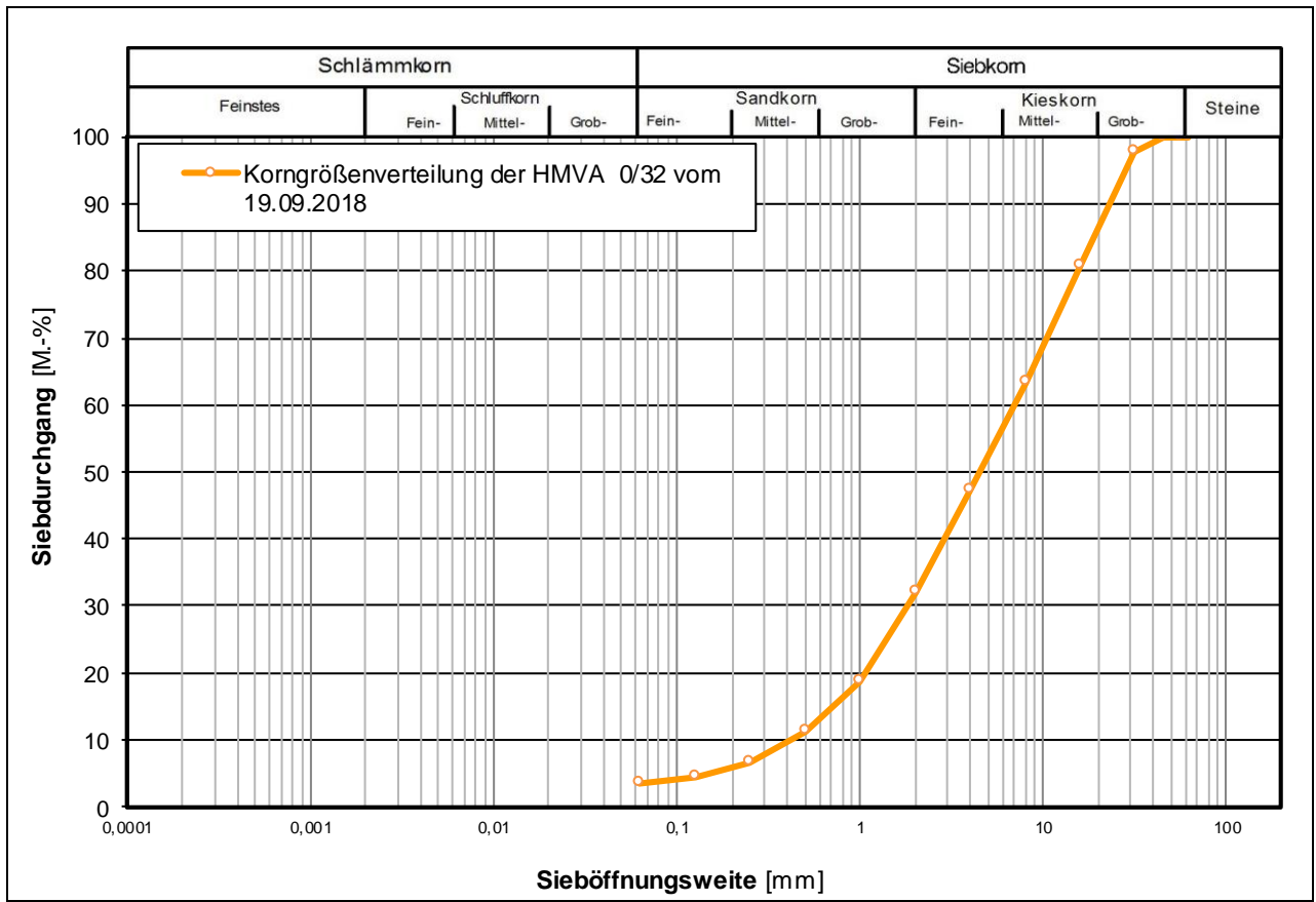
Korngrößenverteilung der untersuchten HMV-Asche 0/32
